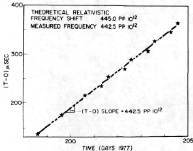
Fig. 20 - Cesium frequency via (T-O) slope
