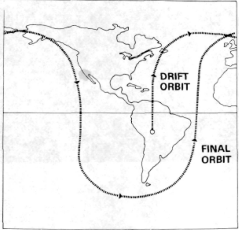
Fig. 5 - NTS-2 drift orbit
